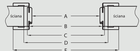
D - wymagana szerokość otworu w murze
