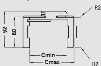
Przekrój ORB 075
