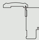
Połączenie opaski z ościeżnicą
