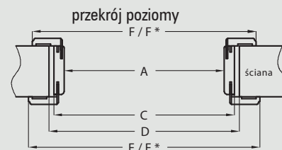
D - wymagana szerokość otworu w murze * dotyczy Tunelu Regulowanego TOP
