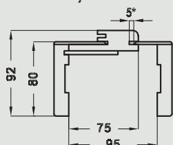
Przekrój ORB 075
